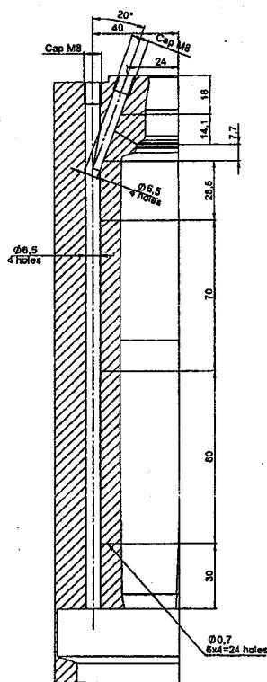
SECTION C-C D-D
